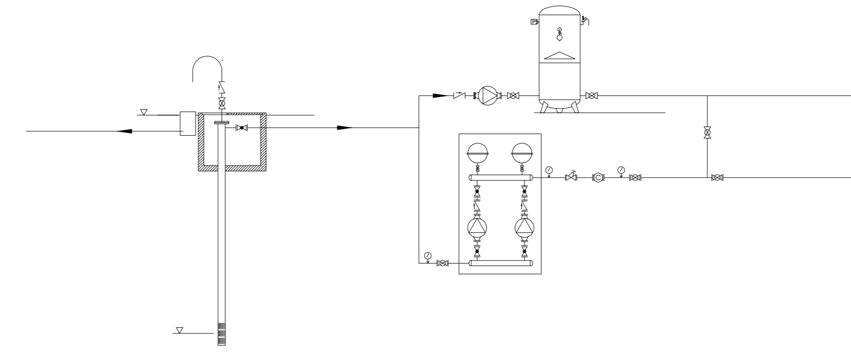
Schema dal pozzo artesiano al vano tecnico
