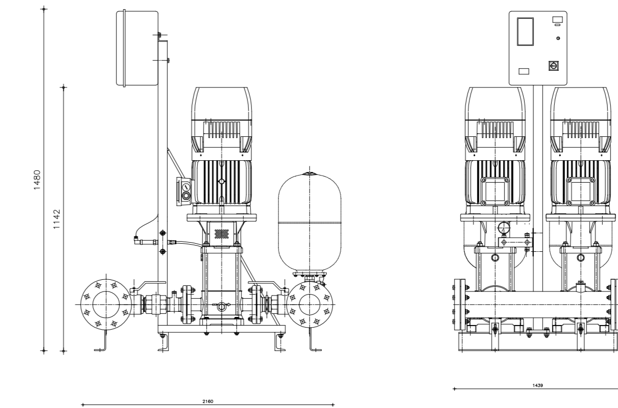
Particolare gruppo di pressurizzazione
