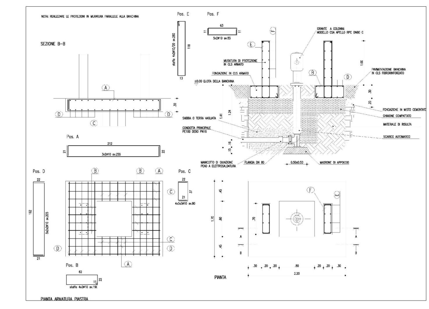
PARTICOLARE IDRANTE SOPRASSUOLO UNI 70 scala 1:20
