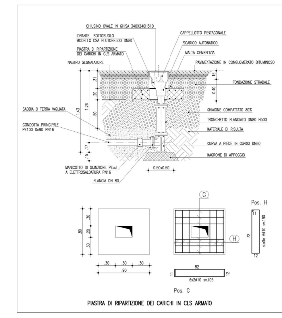
PARTICOLARE IDRANTE SOTTOSUOLO UNI 70 scala 1:20
